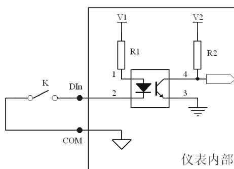
图 3.2 开关量输入接口电路示意图
