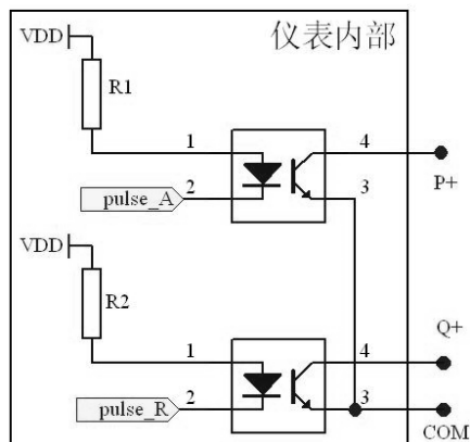
图 3.1 功率脉冲输出接口电路示意图
