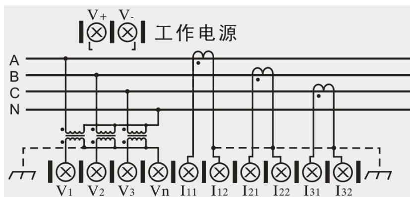
图 5.4 三相四线(带 PT)接线图
