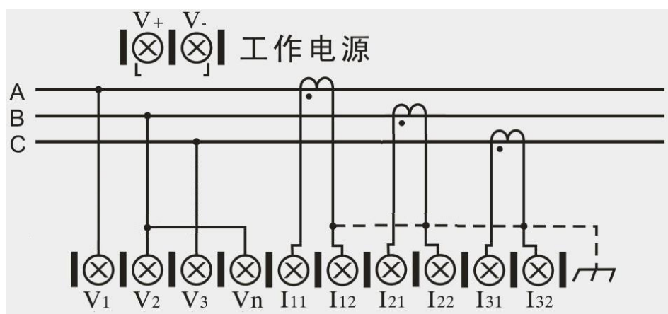
图 5.6 三相三线(无 PT)接线图
