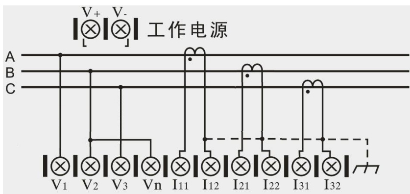
图 5.6 三相三线(无 PT)接线图
